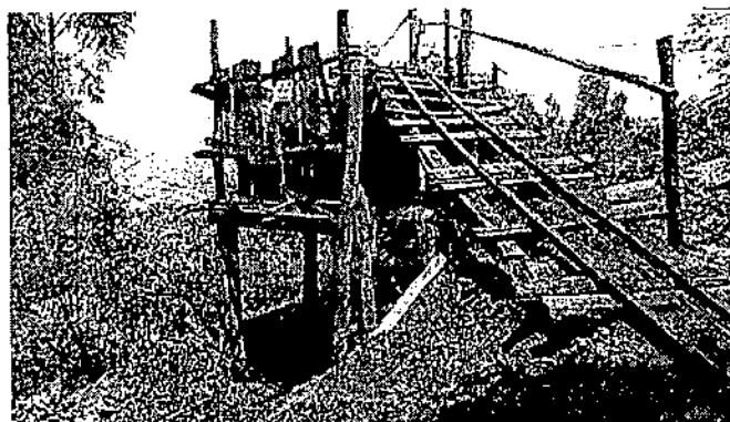
Figura 4. Tolvo de madera en mina La Esmeralda.
