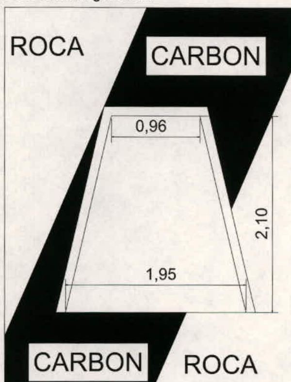
Figura 2 Sostenimiento mina la guevona
