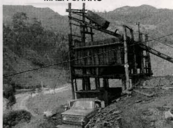
VAGONETA Y TOLVA EN MADERA
