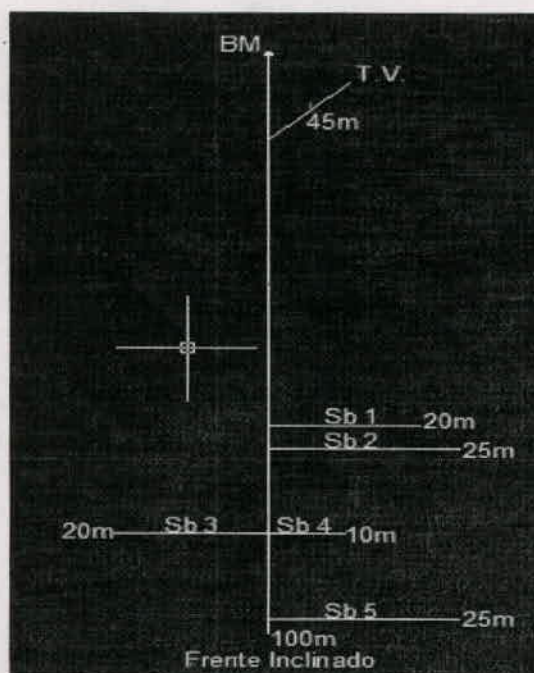
Figura 1. Vista en planta del Inclinado I, operado por el solicitante Luis Enrique Estupiñan Estupiñan
