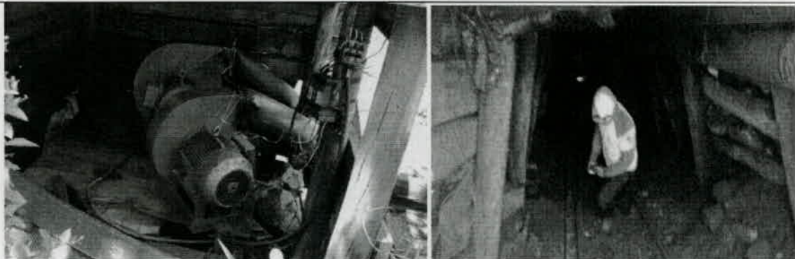
VENTILADORES E INCLINADO, MINA LA MILAGROSA
