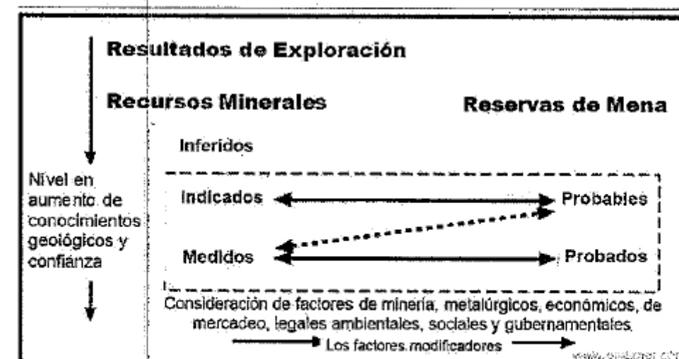
Figura 1: Relación general entre Resultados de Exploración, Recursos y Reservas Minerales.
