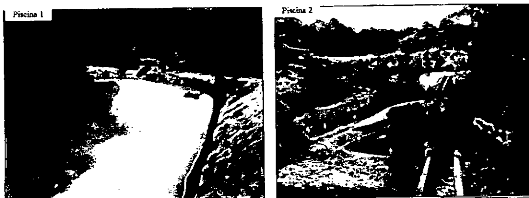
Fotografía 9. Sistema de tratamiento de efluvios. Detalle Piscinas Sedimentación 1 y 2.
