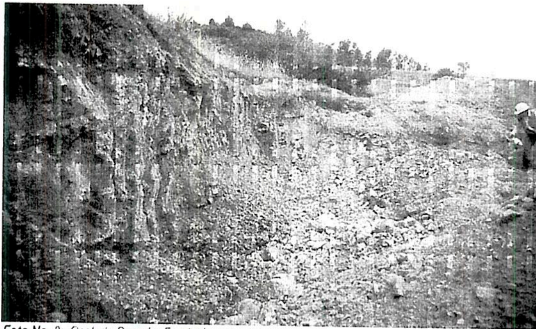
Foto No. 2: Costado Derecho Frente 1- con evidencia de corte y arranque sobre la cara del talud. N: 1.107.266, E: 1.091.283, Z: 2.837 msnm
