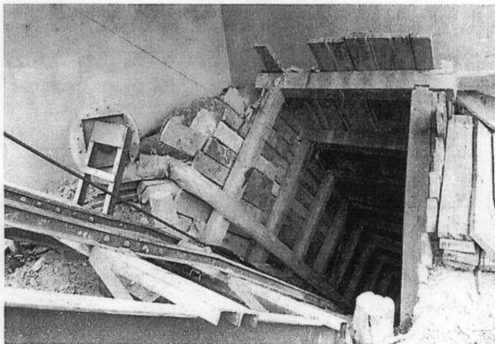
Fotografía No. 7 Bocamina el Salvio Bocamina que se ubica dentro del área del título minero, pero se evidencia que sus labores salen fuera del área del título minero cuenta con un inclinado de aproximadamente de 224 metros con un rumbo N70W y una inclinación de 45 grados, sostenimiento en puerta alemana dente sencillo, separación entre puertas cada metro este inclinado conecta con un nivel con rumbos N40E y S40W cada uno de una longitud aproximada de 100 metros. Coordenadas N 1072409.0, E 1041723.0, Alt 2872
