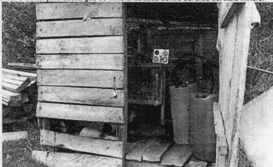
Fotografía No. 4 Compresor de combustible para genera aire a dos martillos neumáticos, ubicados dentro del área del título minero HCE-081.
